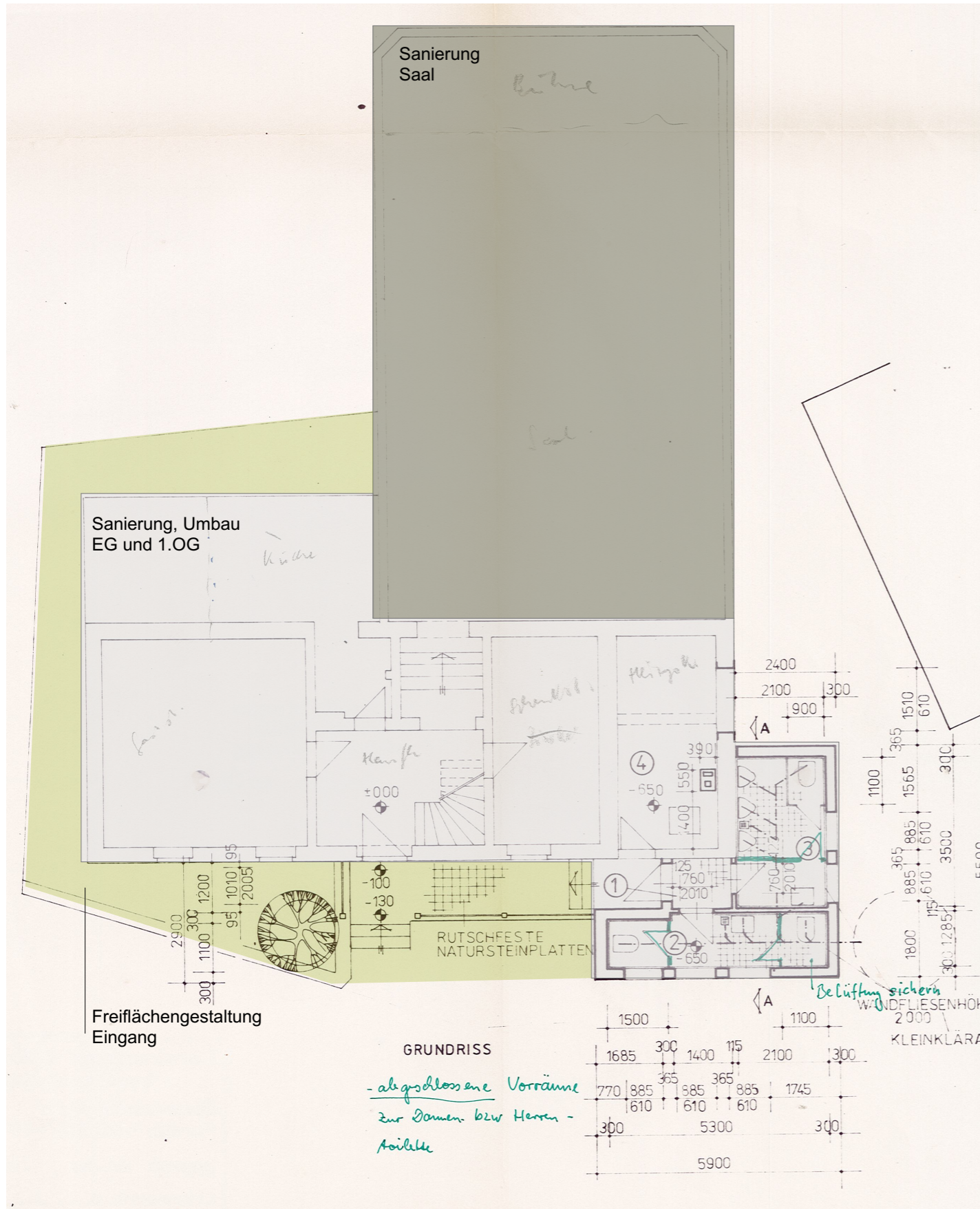
Grundriss
